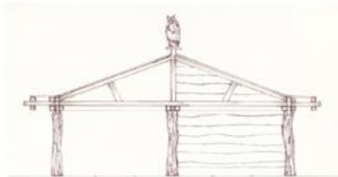
Voor aanzicht uitbouw
